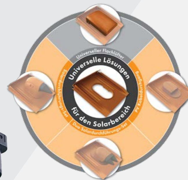
1 Flache Lüfterkappe passend unter Aufdachsolaranlagen 2 Universelle Grundplatte in Standardausführung für flach bis mittel profilierte Dachziegel und Dachsteine, Decklänge 310 - 350 mm 3 Adapter DN 110 und DN 125 für verschiedene Nennweiten
